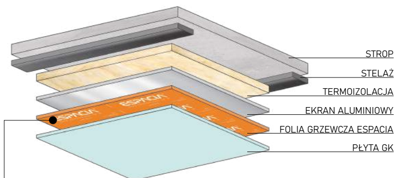
SYSTEM GRZEWczy SUFITOWY
